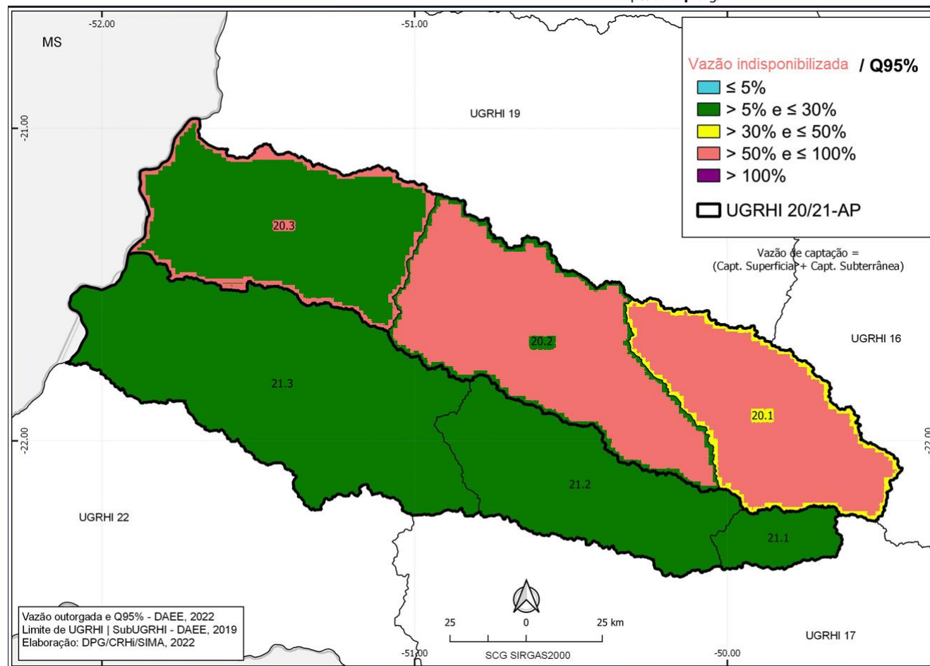
Figura 9 - Vazão indisponibilizada na Bacia em função de outorgas e licenciamentos
