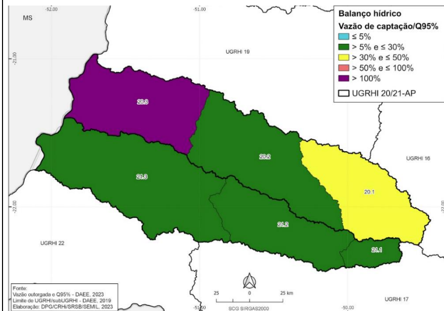
Figura 7 - Relação entre captação e a vazão disponível Q 95%
