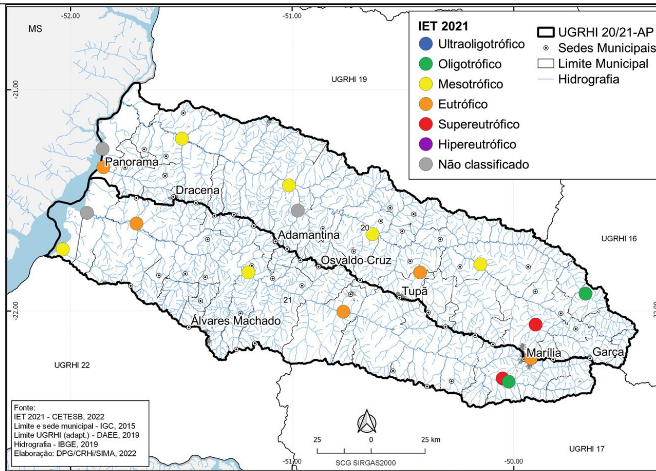
Figura 15: IET das UGRHIs 20 e 21.
