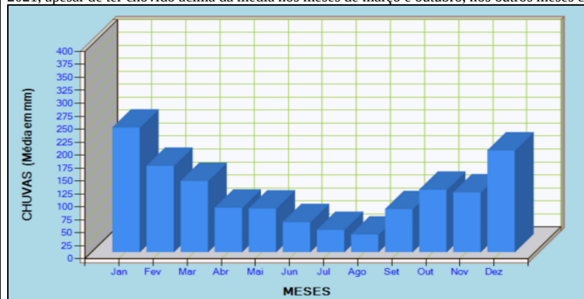
Pluviograma da média mensal de 1971 a 2015 da UGRHI 20 e 21 - Fonte: DAEE (2015).
