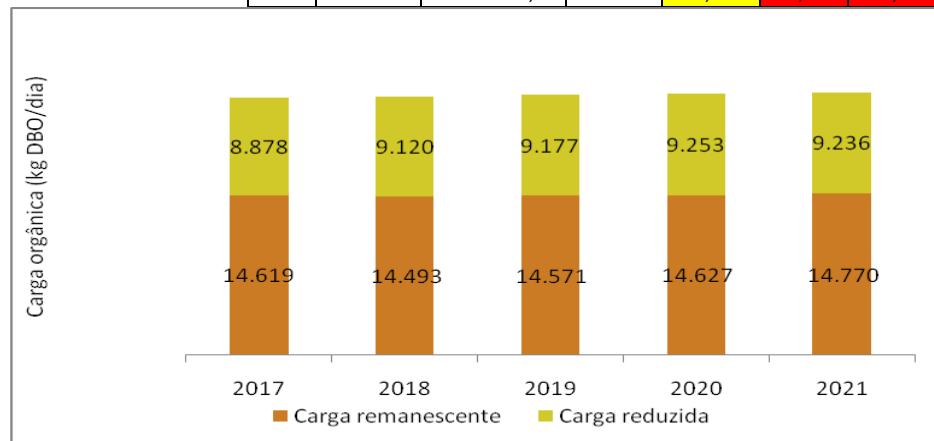
Figura 13 - Carga remanescente da Bacia do Peixe
