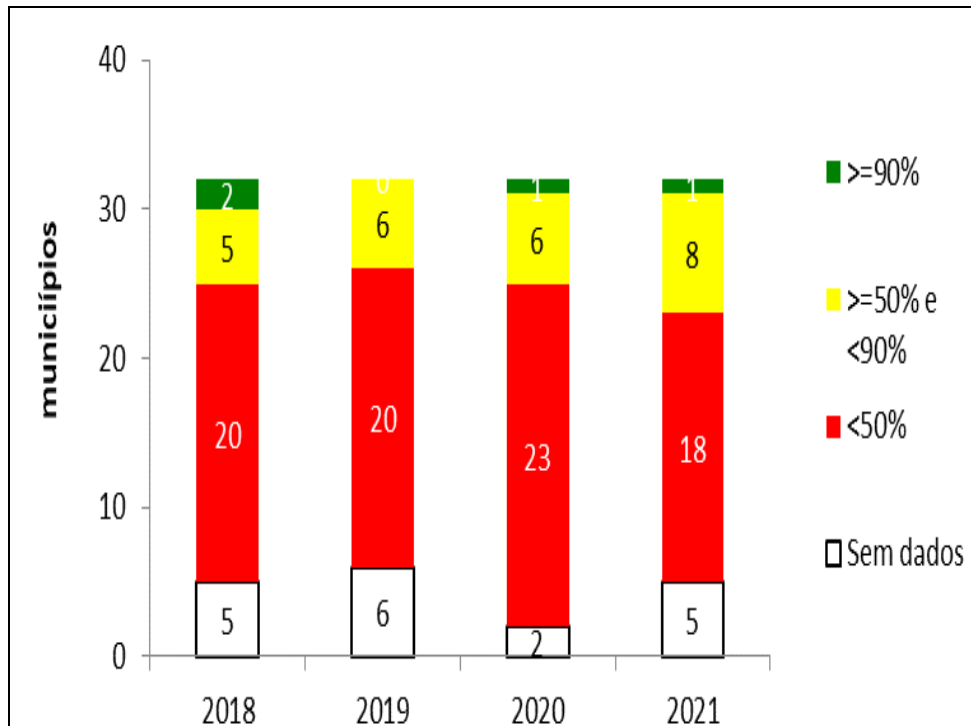
Figura 18 - Indicação de taxa de cobertura de drenagem urbana subterrânea inferior a 50% para a maioria dos municípios das UGRHIs 20 e 21
